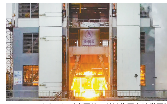
试车现场。(中国航天科技集团六院供图)
